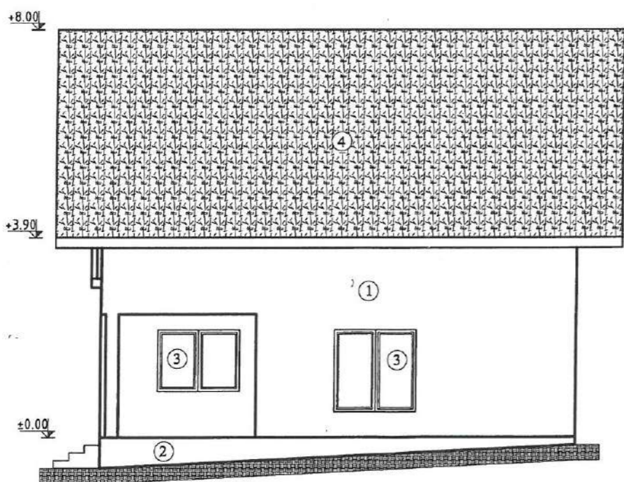
FATADA LATERALA D-D
