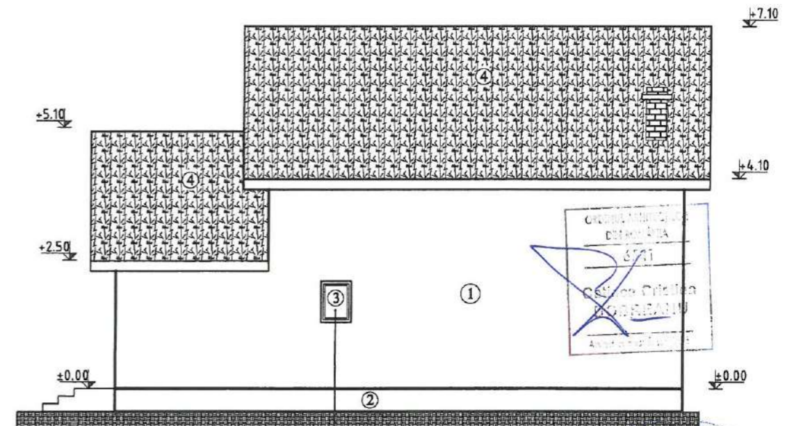
FATADA POSTERIOARA C - C
